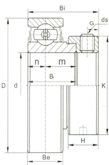
CSA 200 (light-duty) Cylindrical O. D.
