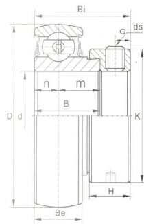
SA 200 (light-duty) Spherical O. D.
