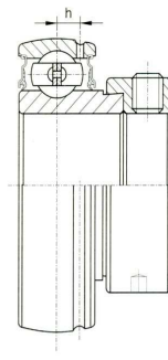
SA 200G Relubricatable type
