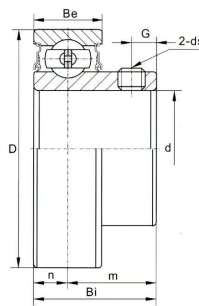
CSB 200 (light-duty) Cylindrical O. D.
