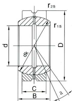
GE...ES
