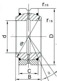
GE...ES-2RS
